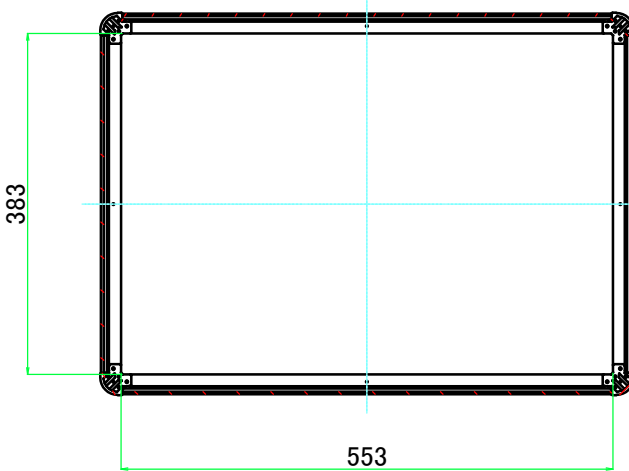
C-C ( 1 : 8.5 )
